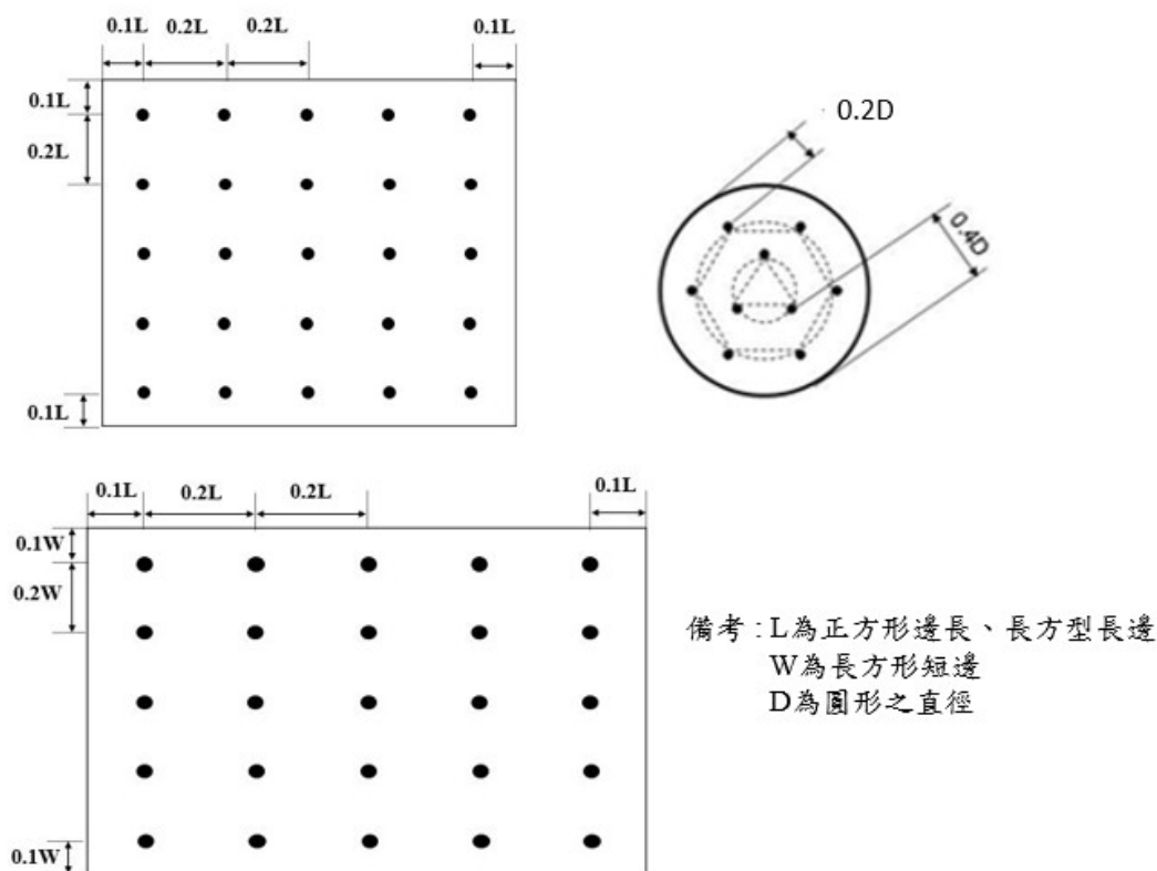
圖1 輝度均勻度量測點示意圖
