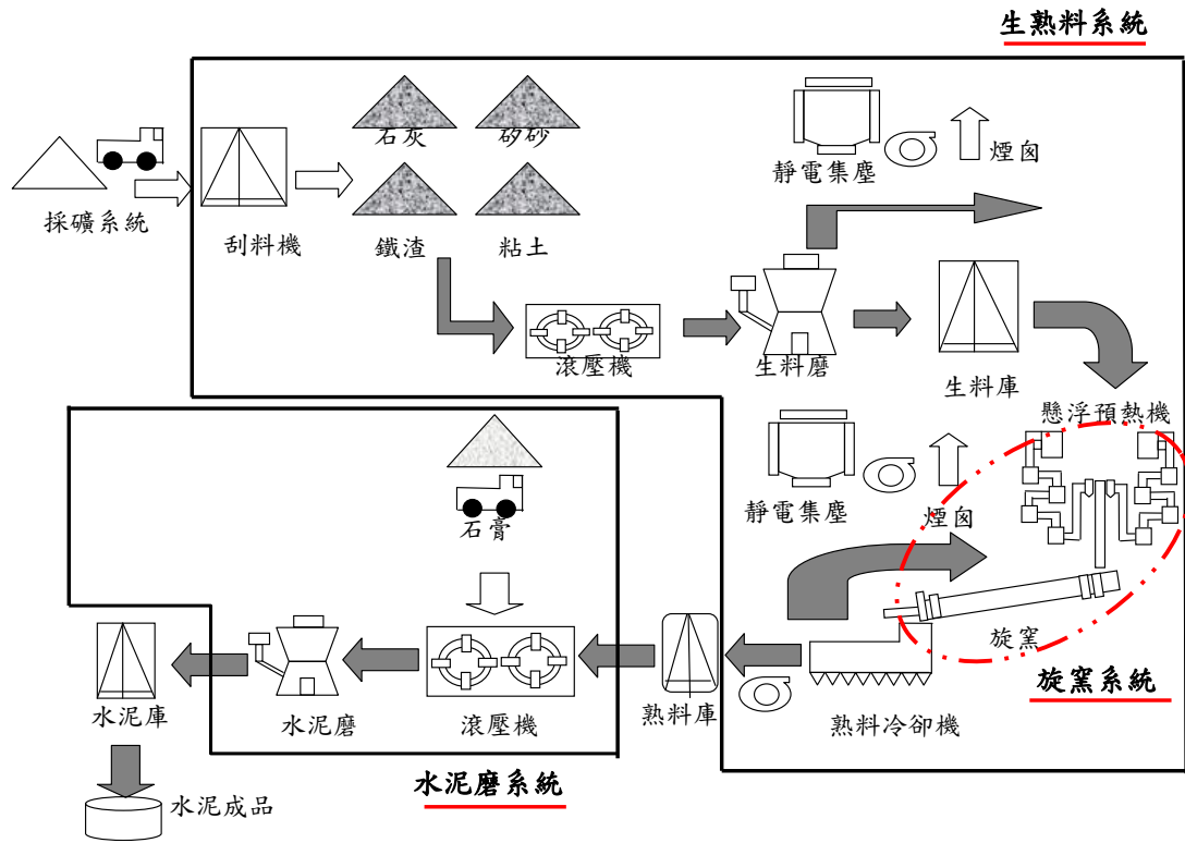
圖1 水泥製造業製程設備系統範圍界定圖
