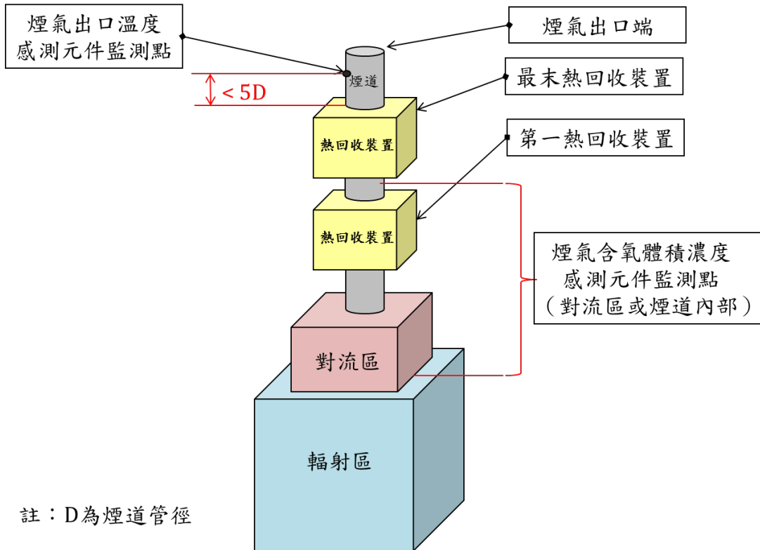
圖二 加熱爐或裂解爐（已設置熱回收裝置）煙氣含氧體積濃度及煙氣出口溫度之監測點
