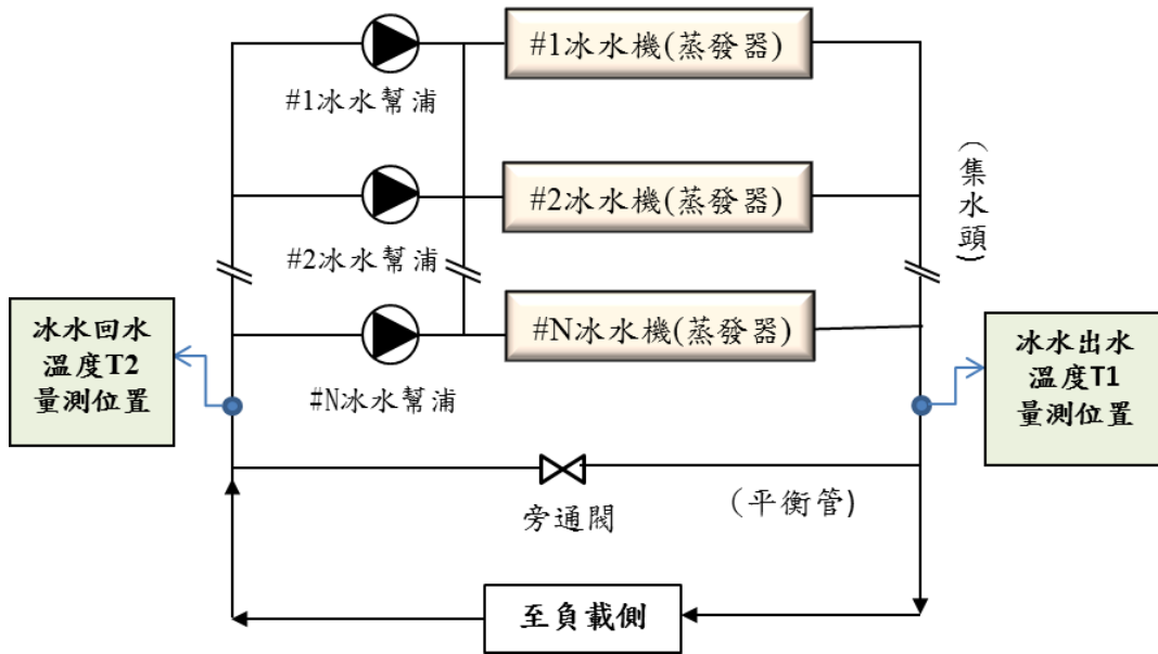
圖三 冰水機蒸發器冰水出水、回水溫度差量測位置
