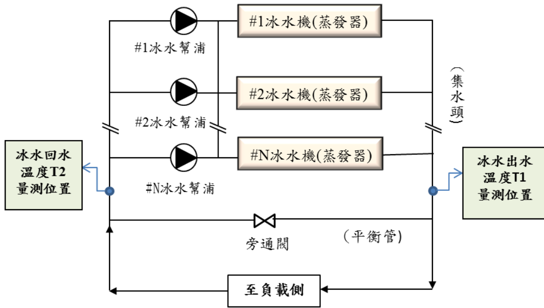
圖一 冰水機冰水出水、回水溫差量測位置
